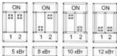
Рис. 9. Положение рычагов переключателя мощности.
