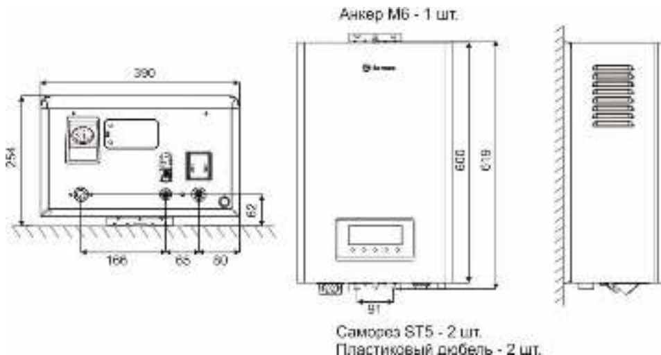
Рис. 6. Монтажные размеры
