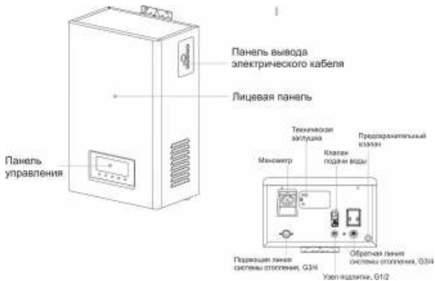
Рис. 1. Конструкция изделия
